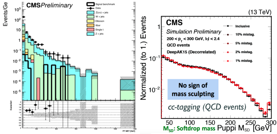
Figura 2: Esquerda: distribuição da E_T^{miss} em uma região de controle ("0 b-tagged signal region") do conjunto de dados de 2016 para dados reais e simulação. Direita: distribuição da massa "Puppi SoftDrop" (uma medida da massa do jato hadrônico) tanto de modo inclusivo (preto) como com diferentes pontos de operação do algoritmo identificador de jatos (tons de vermelho).
