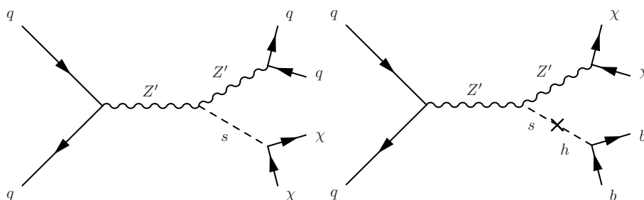
Figura 1: Diagramas de interesse para produção do Higgs escuro no LHC.
