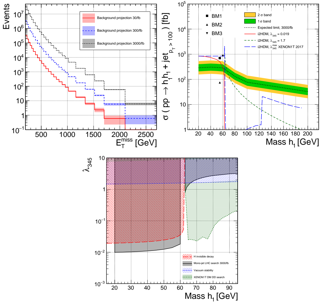
Figura 5: Alto, esquerda: projeção do fundo de Modelo Padrão para a busca por matéria escura no contexto do modelo i2HDM, para os cenários de 30, 300 e 3000 fb ^{-1} tomados com o detector CMS. Alto, direita: limite esperado para a mesma situação – as linhas vermelha cheia e verde pontilhada representam a seção de choque de diferentes possíveis configurações do modelo i2HDM; a linha azul tracejada representa a máxima seção de choque possível para o modelo, em conjunto com os resultados do experimento XENON 1T [23]. Baixo: reinterpretação dos limites no espaço de parâmetros do modelo i2DHM, m_{h_1} \times \lambda_{345} .
