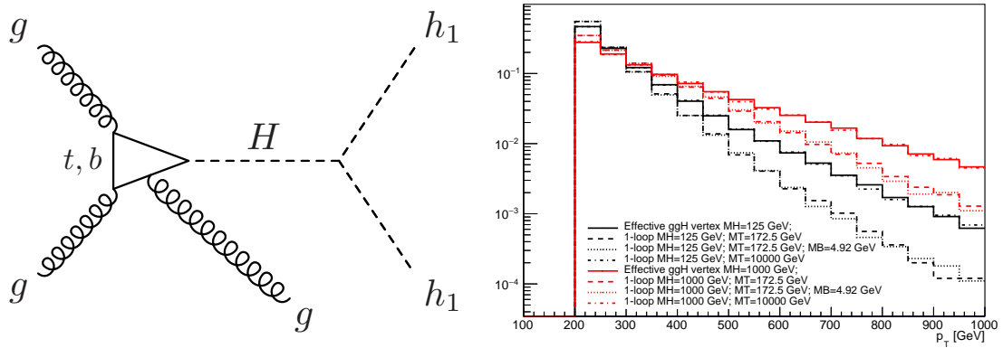
Figura 4: Esquerda: expansão do loop do quark top, relevante para o processo pp \rightarrow h_1 h_1 + \text{jatos} do modelo i2HDM, onde h_1 é uma nova partícula de Higgs que assume o papel de matéria escura. Direita: modificação do espectro de p_T do bóson de Higgs com as correções da expansão supracitada. O efeito das correções é tornar o espectro muito mais suave, o que diminui fortemente as chances de detecção do processo.
