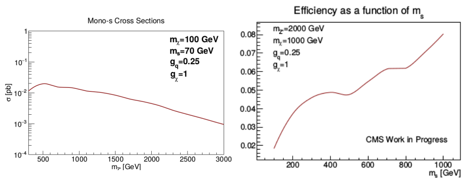
Figura 3: Esquerda: seção de choque para o processo pp \rightarrow \chi\chi s , calculada para os parâmetros do modelo de Dark Higgs mostrados no gráfico, para colisões pp com \sqrt{s} = 13 TeV. Direita: eficiência de seleção de eventos de sinal, seguindo proposta de critérios de seleção sugerida em [26].
